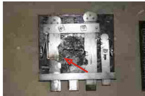
Blockierung des unteren Schlüssels vor Auslösung des Schnappmechanismus durch Form der Riegelaussparung
